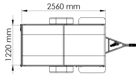
Plancher et pont en tôle alu à damier
