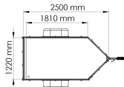
Ridelles en tôle galvanisée à chaud
