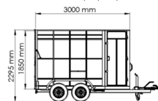
Côtés bois marron Contreplaqué ép.15mm lisse
