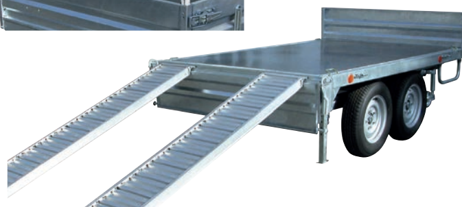
Option rampes de montée logées sous la benne
