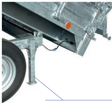
Pieds de béquillage arrière
